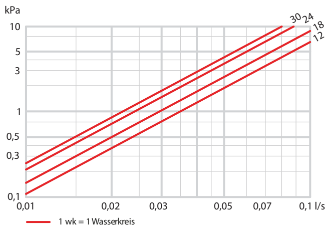
Diagramm 4 Druckabfall Heizwasser, ActiveBeam2 M-1 und ML-1
