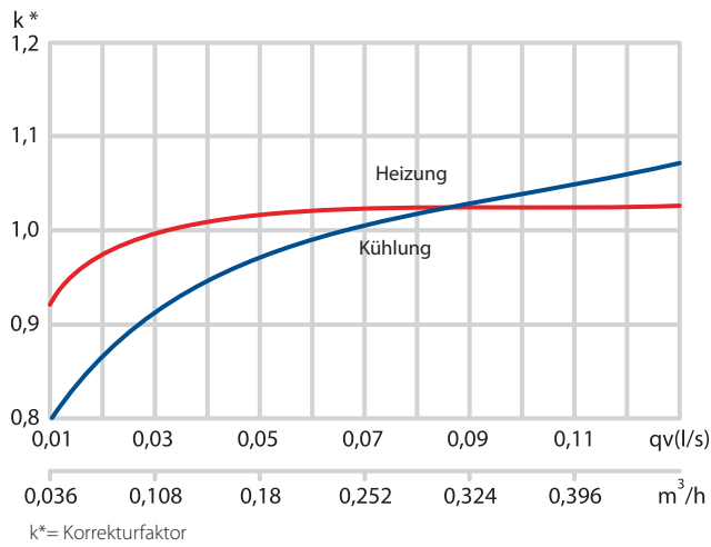
Diagramm 1 Korrekturfaktor K* für den Wasservolumenstrom
