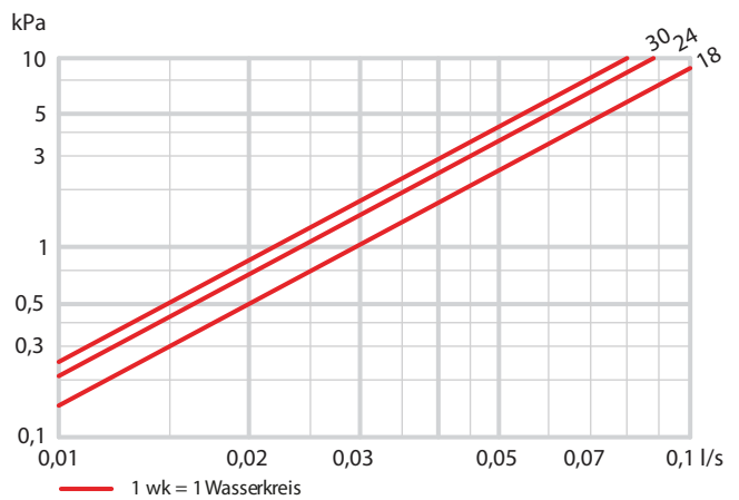
Diagramm 5 Druckabfall Heizwasser, ActiveBeam2 M-2 und ML-2
