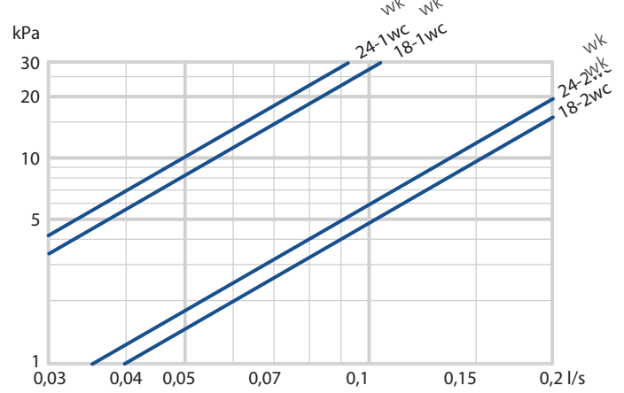
Diagramm 2 Druckabfall Kühlwasser
